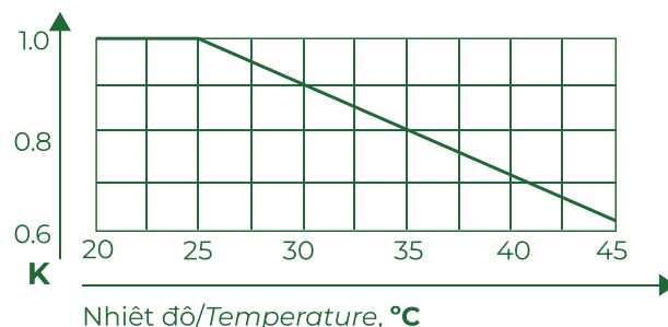
Hình 1: Biểu đồ K đối với ống PVC-U
