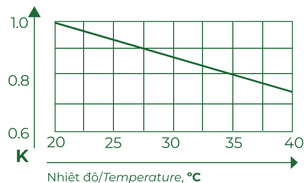
Hình 1: Biểu đồ K đối với ống HDPE
